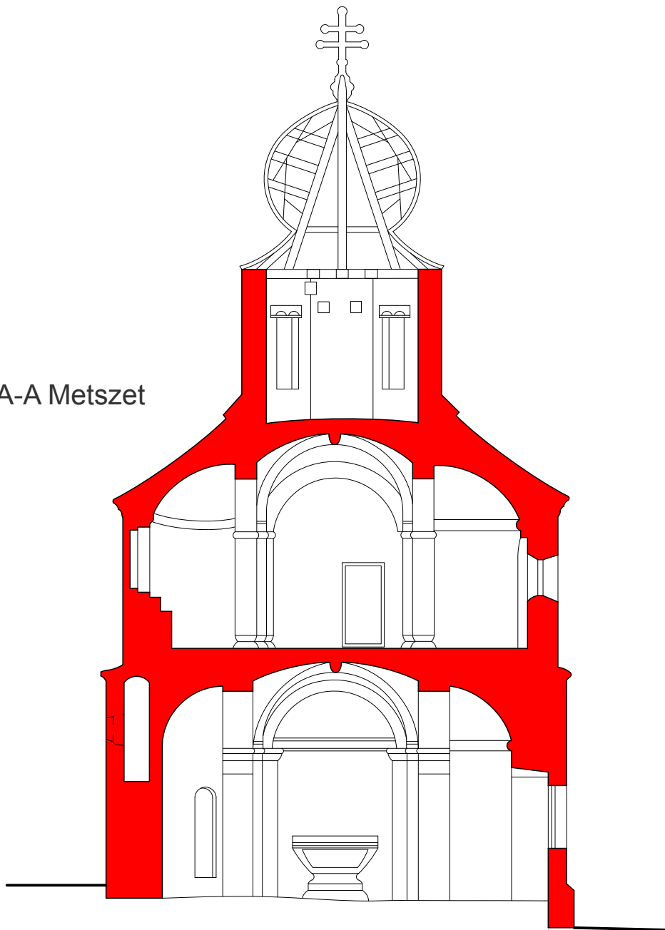
A templom keresztmetszete és alaprajza
